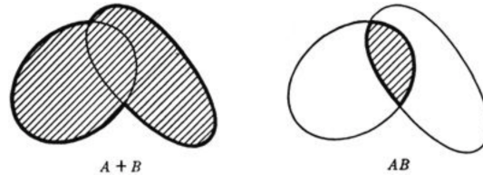
Hình 2.19: Hợp và giao của các tập hợp
