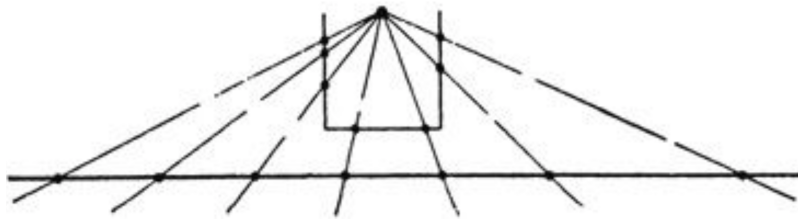
Hình 2.13: Sự tương ứng một-một giữa các điểm của một khoảng (bị gấp lại) với các điểm của đường thẳng
