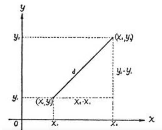
Hình 2.7: Khoảng cách giữa hai điểm
