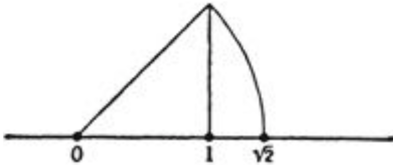
Hình 2.3: Cách dựng số \sqrt{2}
