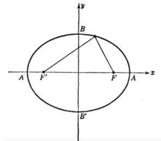
Hình 2.9: Elip với các tiêu điểm
