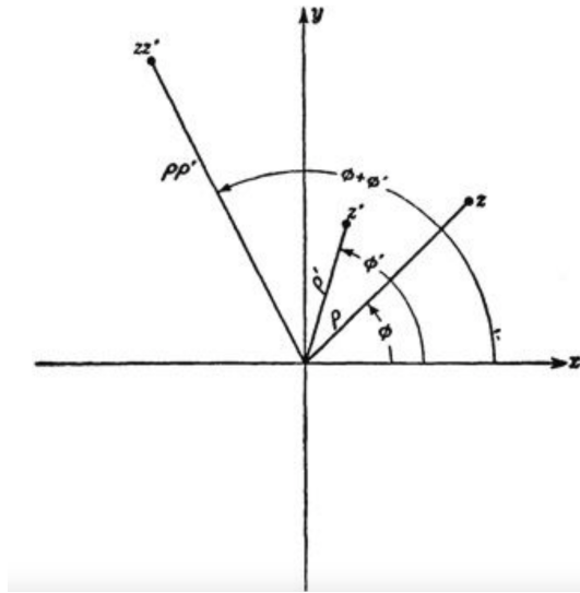
Hình 2.17: Phép nhân các số phức: cộng các argumen, nhân các modulo
