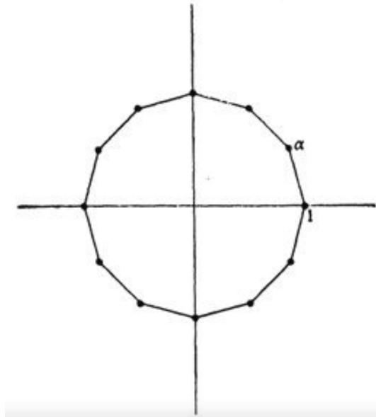
Hình 2.18: Mười hai nghiệm của lũy thừa bậc 12 của đơn vị
