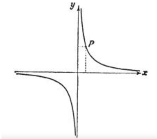
Hình 2.11: Hypebon cân diện tích hình chữ nhật xác định bởi điểm P(x;y) bằng 1
