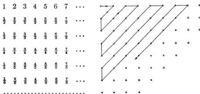
Hình 2.12: Đánh số các số hữu tỉ
