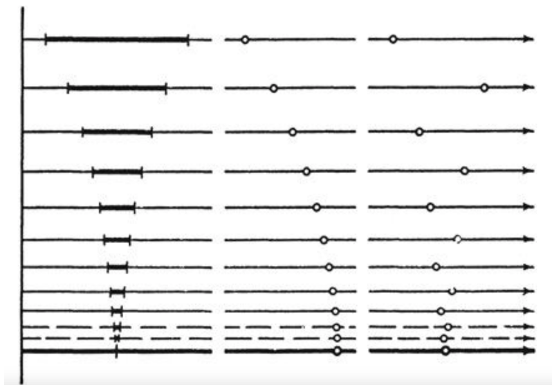
Hình 2.4: Các đoạn thắt. Giới hạn của các dãy
