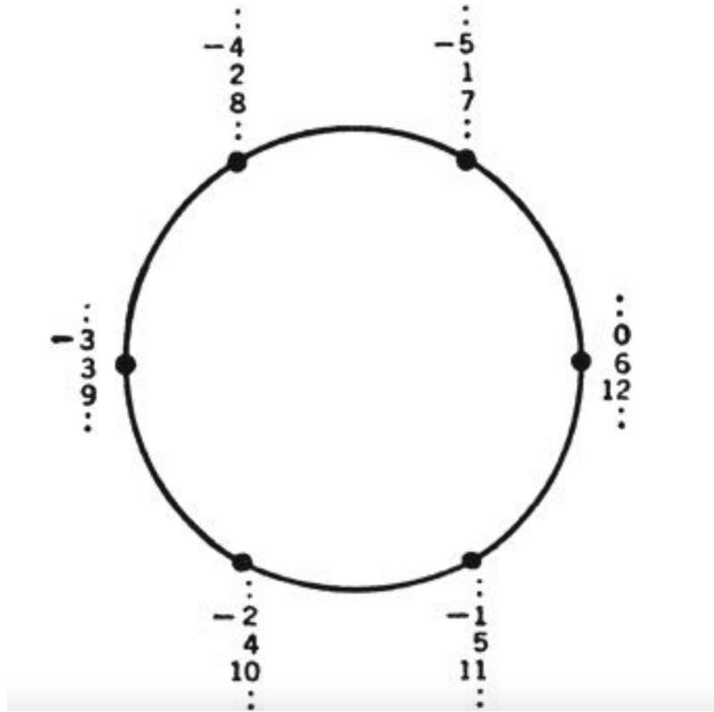
Hình 1.9: Biểu diễn hình học các số nguyên theo modulo 6
