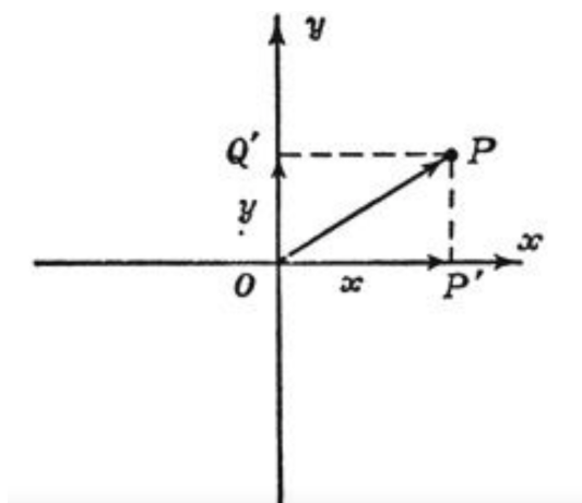
Hình 2.5: Tọa độ vuông góc của một điểm.
