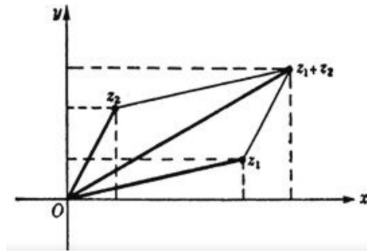
Hình 2.16: Phép cộng các số phức theo quy tắc hình bình hành
