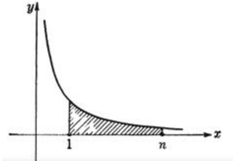
Hình 1.7: Diện tích miền có gạch ở dưới hypebol xác định hàm số \ln(n)
