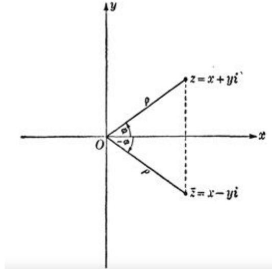
Hình 2.15: Biểu diễn hình học của số phức. Điểm z có tọa độ vuông góc x, y
