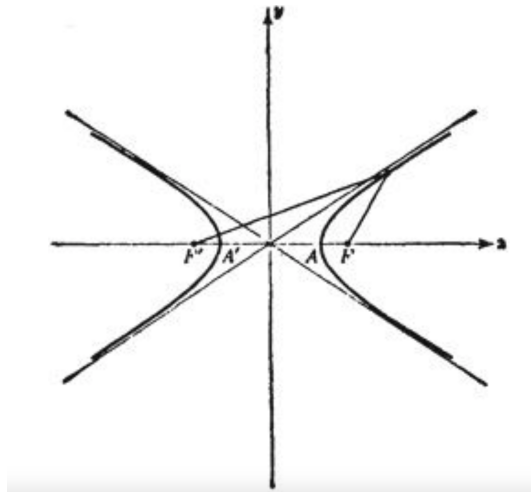
Hình 2.10: Hypebon với các tiêu điểm
