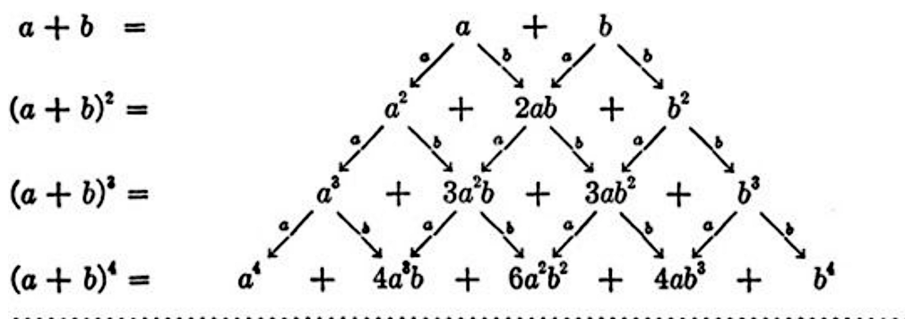
Hình 1.5: Sơ đồ định lý nhị thức
