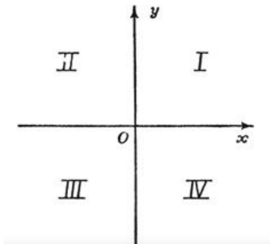
Hình 2.6: Bốn góc phần tư.
