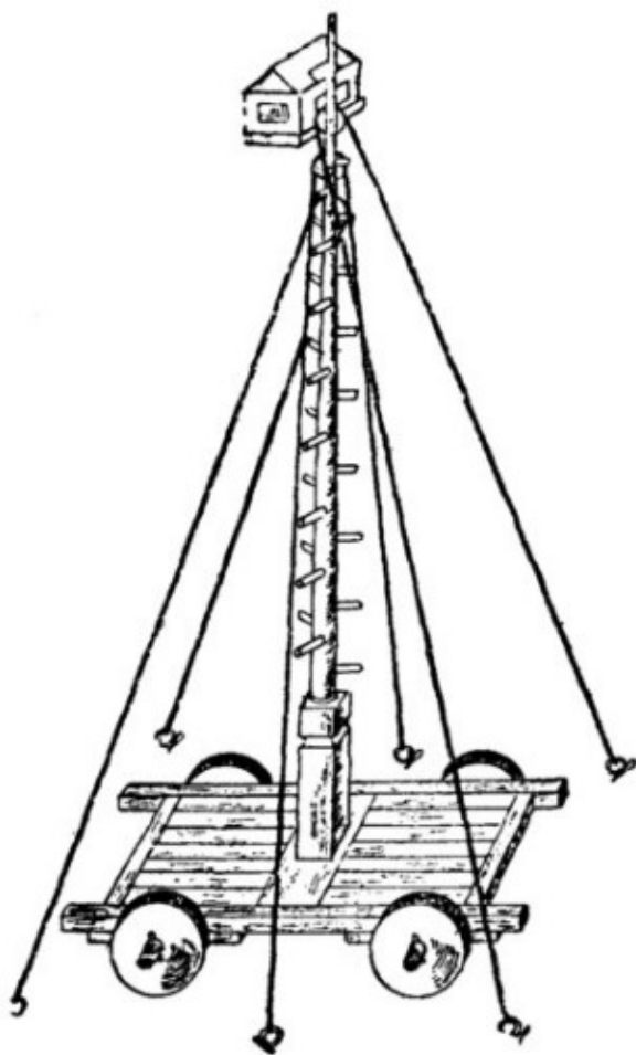
Hình 40. Xe vọng lâu
